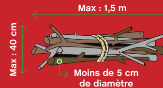
BRANCHES ATTACHÉES EN BALLOT
